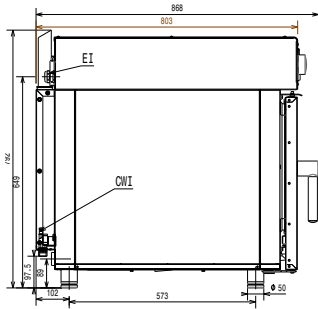
Oldalnézet
